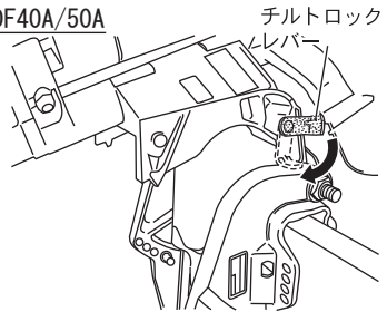
DF40A/50A
